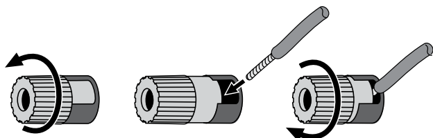
1. Skru hættan løs 2. Isæt afisoleret ledningsende 3. Skru hættan fast
